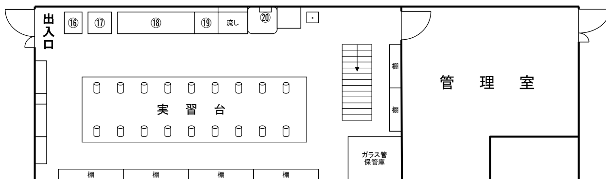
2階
