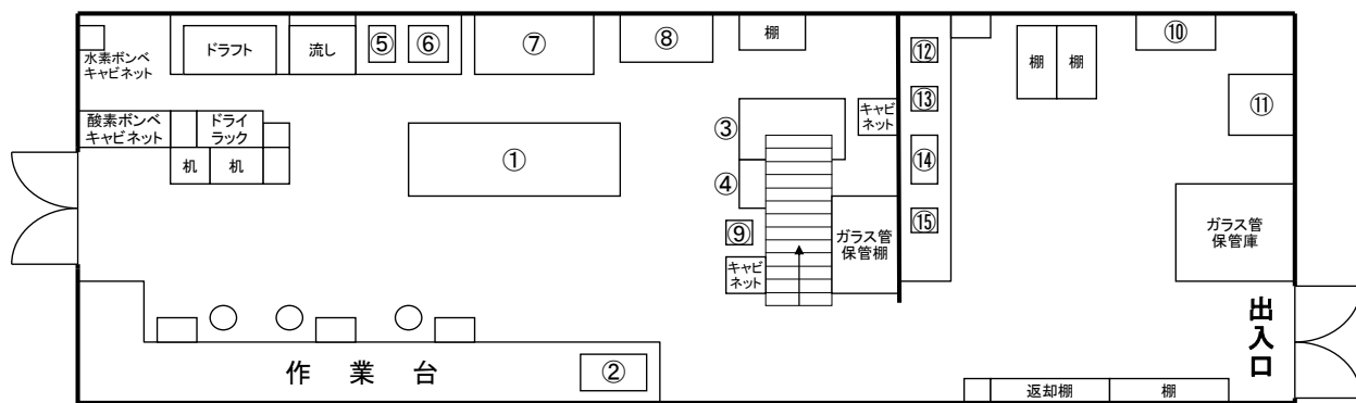
1階
